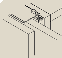
Connector 55 mm: nicchia per una anta roto-rientante.
