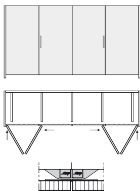
Centraggio anta con rampa di fissaggio.
