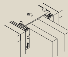
Connector 110 mm: nicchia per due ante roto-rientanti.
