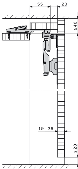
Centraggio anta con centraggi magnetici.
