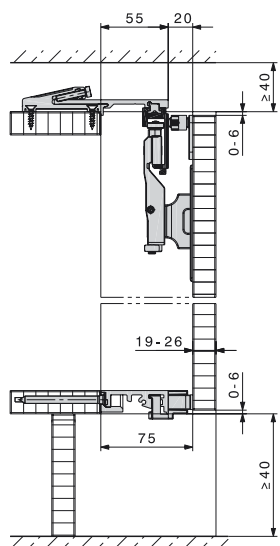
Centraggio anta con rampa di fissaggio.
