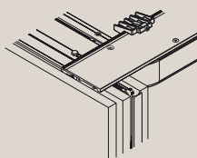
Componente della guarnitura HAWA-Folding Concepta 25: profili di collegamento laterale e al corpo come ingegnoso ausilio al montaggio con frontali davanti al corpo dell'armadio.
