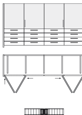
Centraggio anta con centraggi magnetici.
