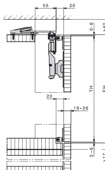
Centraggio anta con centraggi magnetici.
