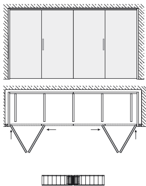
Centraggio anta con centraggi magnetici.
