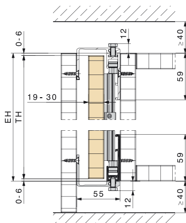
HAWA-Concepta 25/30 con Connector 55 mm.
